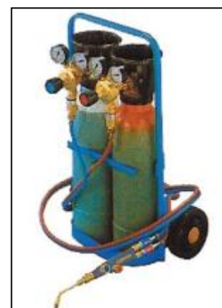
Saldatura portatile ossigeno acetilene
