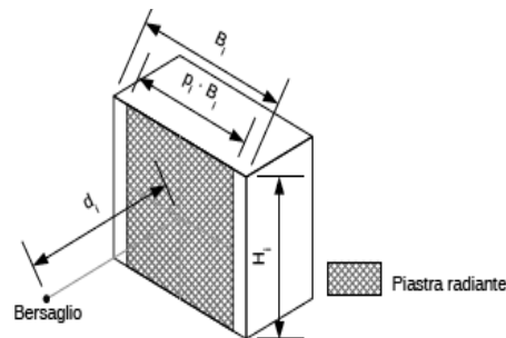
Illustrazione S.3-5 Schematizzazione della piastra radiante
